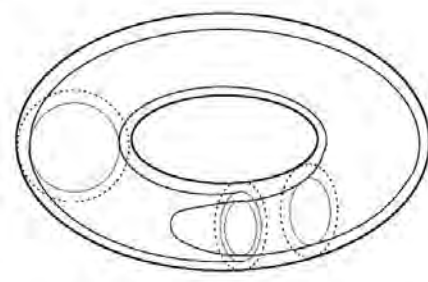
図2: ソリッドトーラス ( D^2 \times S^1 , ドーナツ) のReeb 葉層の葉 (平面と同相)
