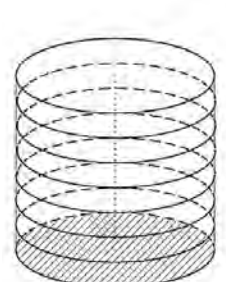
図1: D^2 \times I の積構造
